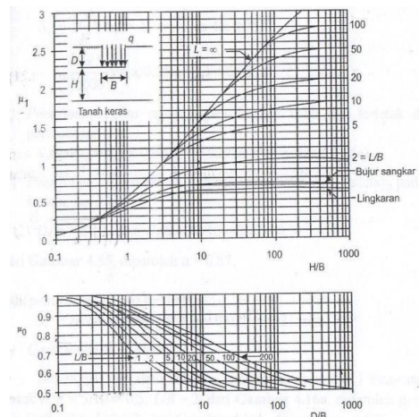
Gambar 2.2. Grafik hubungan \mu_i , \mu_0 , kedalaman fondasi ( D_f ), dan lebar fondasi ( B ).
