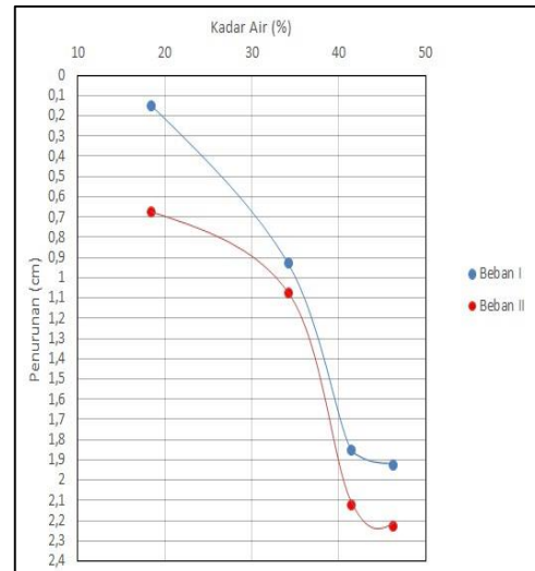
Gambar 4.6 Hasil Grafik Perbandingan Antara Kadar Air dengan Penurunan Fondasi
