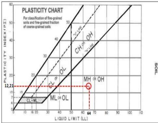
Gambar 4.2. Klasifikasi Tanah Desa Kalikayen Metode USCS
