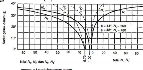
Gambar 2.1. Hubungan \phi dan N_\gamma , N_c , N_q . (Sumber: Hardiyatmo, 1996).
