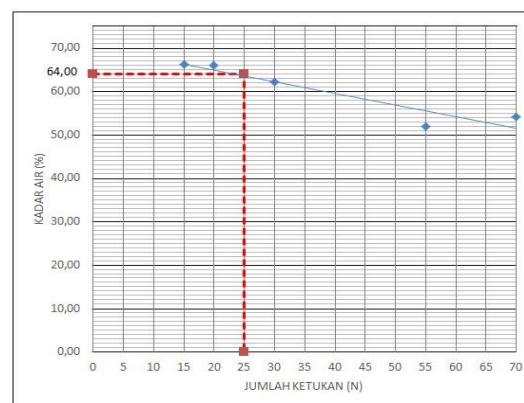
Gambar 4.1 Grafik Uji Batas Cair Tanah Desa Kalikayen
