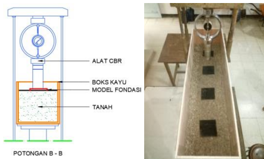
Gambar 3.4 Ilustrasi Pengujian di Laboratorium
