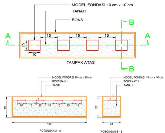
Gambar 3.3 Permodelan Box Wadah dan Fondasi
