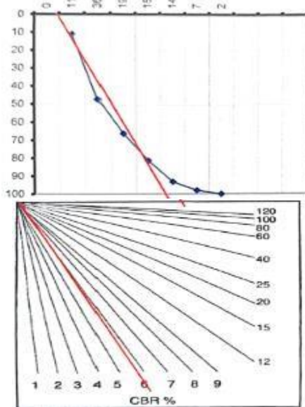
Gambar 4.5 Grafik Pengujian DCP Pada Tanah Desa Kalikayen
