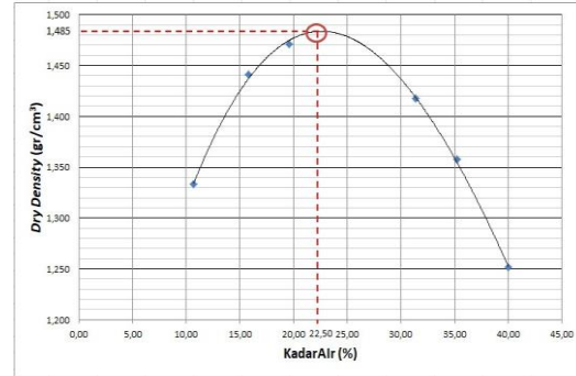
Gambar 4.3 Grafik Uji Kompaksi Tanah Desa Kalikayen
