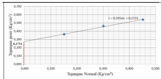
Gambar 4.4 Grafik Perbandingan Antara Tegangan Normal dan Tegangan Geser
